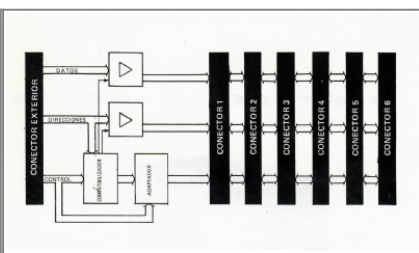
Diagrama de bloques del CR-401
