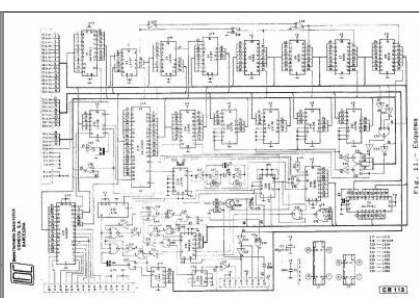
Diagrama electrónico del CR-113
