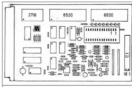
Diagrama del CR-120
