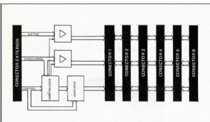
Diagrama de bloques del CR-401
