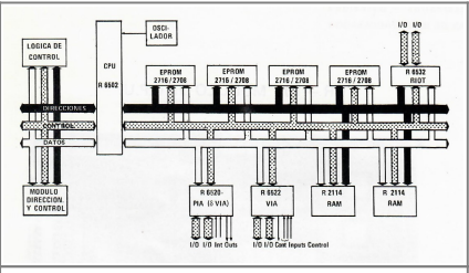
Diagrama de bloques del CR-101
