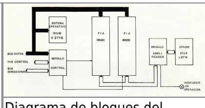
Diagrama de bloques del CR-108
