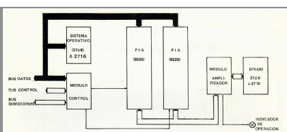
Diagrama de bloques del CR-108
