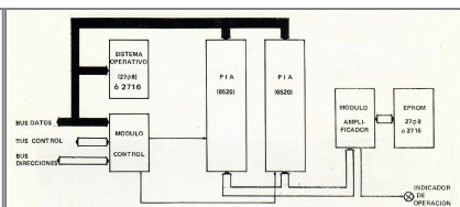
Diagrama de bloques del CR-108
