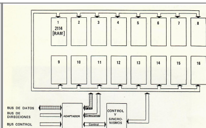
Diagrama de bloques del CR-106
