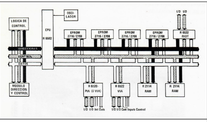
Diagrama de bloques del CR-101
